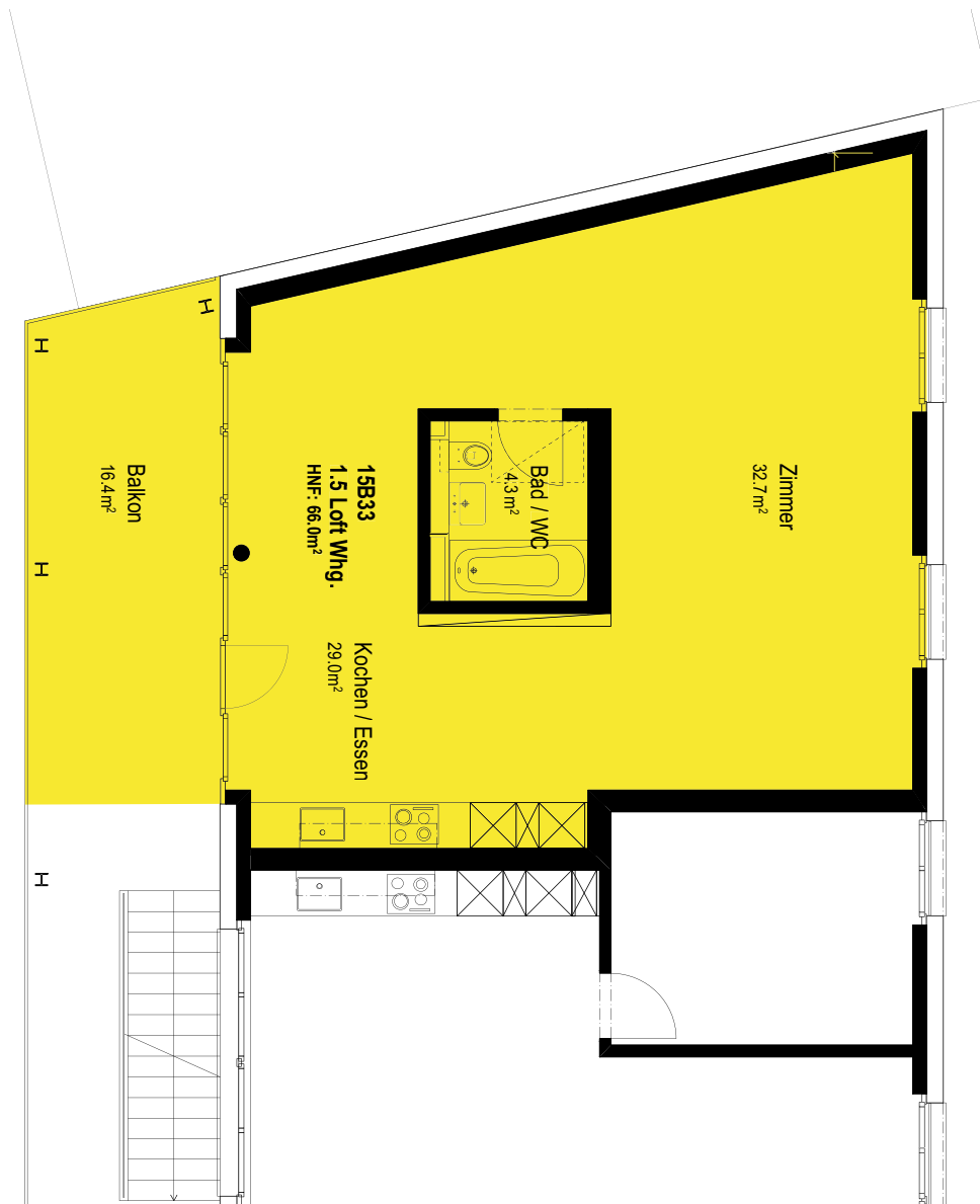
Grundriss 1:100
